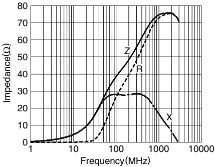
MMZ1005Y400C
