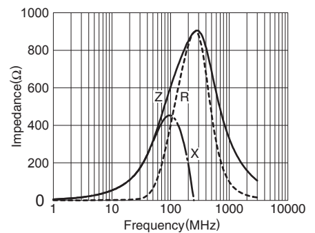
MMZ0603Y601C
