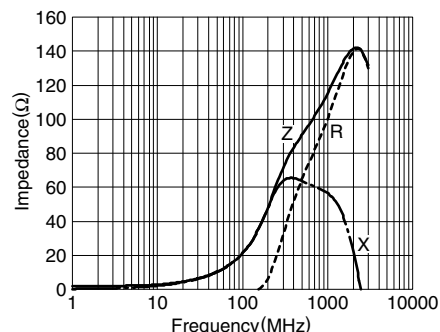
MMZ1608D220C
