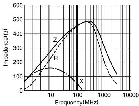
MMZ1608R150A
